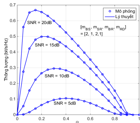
Hình 6. Khảo sát thông lượng hệ thống theo \alpha
