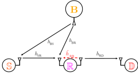
Hình 1. Mô hình hệ thống chuyển tiếp song công thu thấp năng lượng
