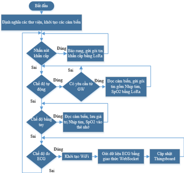
Hình 5. Lưu đồ thuật toán tại Sensor Node
