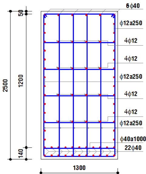
Hình 3. Mặt cắt bố trí cốt thép dầm theo 2DSTM
