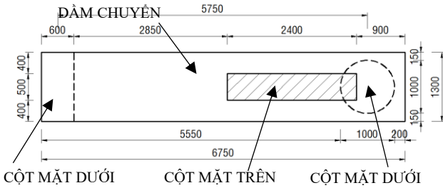
Hình 1. Các đặc trưng kích thước dầm chuyển đỡ cột
