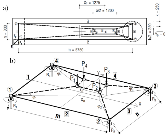
Hình 4. a) Đặc trưng kích thước mô hình giàn ảo không gian b) Mô hình giàn ảo không gian dầm chuyển đỡ cột
