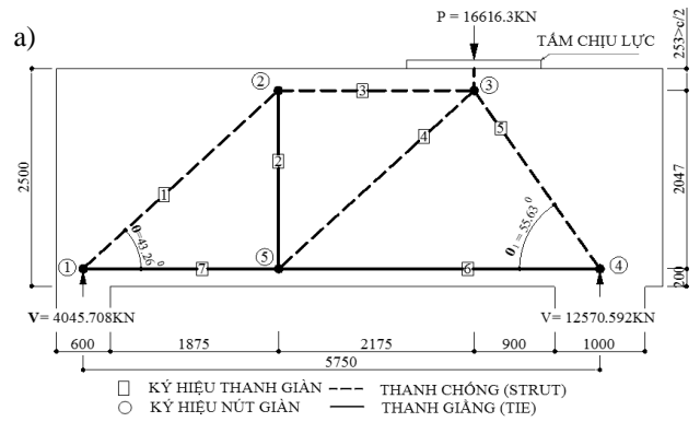
Hình 2a. Mô hình giàn ảo phẳng dầm chuyển đỡ cột
